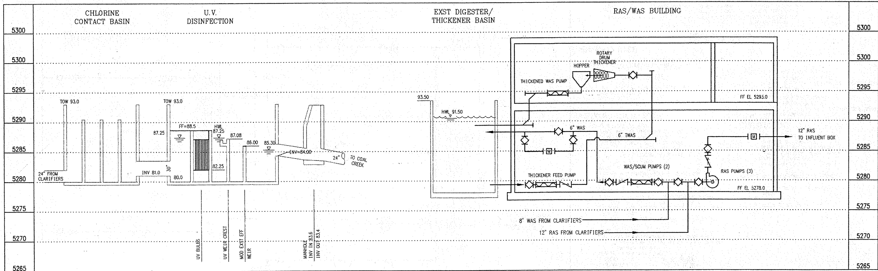
HYDRAULIC PROFILE 1"=5'-0" VERT
