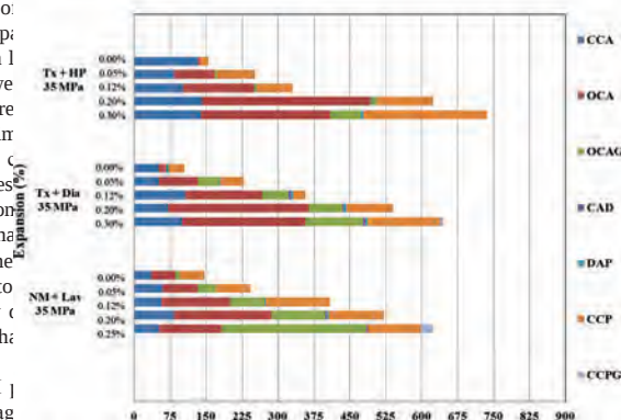
(b) 35 MPa mixtures
